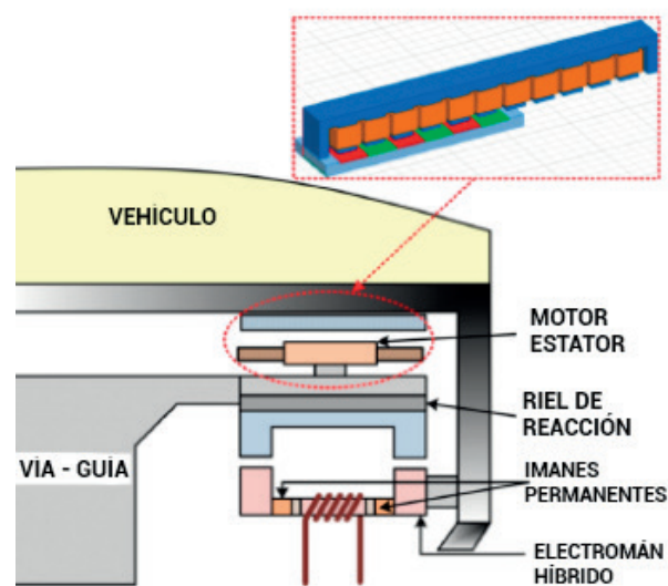
Figura 2. Sistema HEMS
