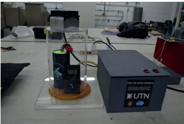
Figura 4. El dispositivo de ensayo de vacío térmico en el Laboratorio de Aerodinámica y Fluidos (LAF) de la UTN FRH
